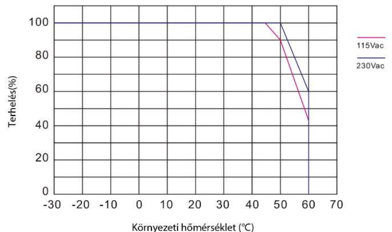
Hőmérsékleti-Terhelési görbe
