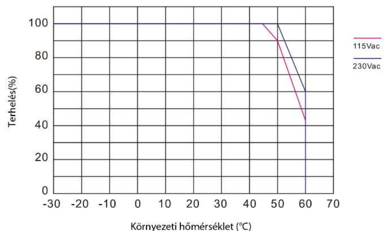
Hőmérsékleti-Terhelési görbe
