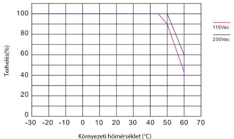
Hőmérsékleti-Terhelési görbe
